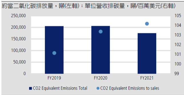
圖 13：碳排量
