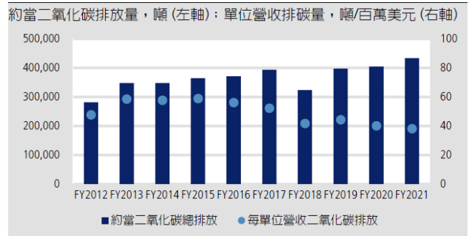
圖 21：碳排量
