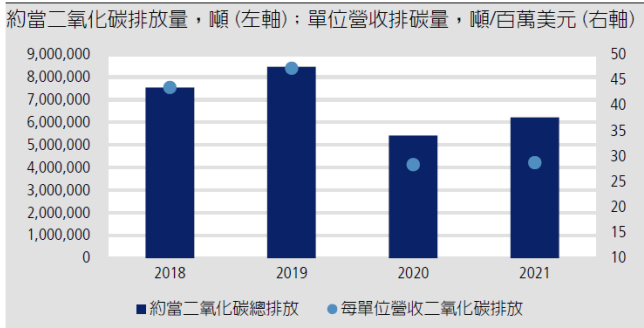
圖 16：碳排放量
