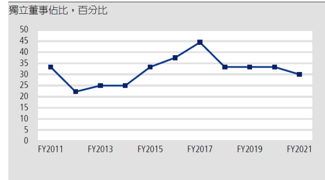
圖 18：獨立董事
